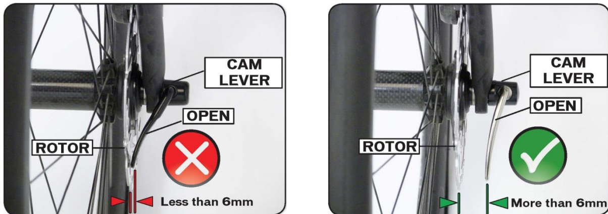
Figura 1. Alavanca de quick-release com potencial de contato Figura 2. Alavanca de quick-release com abertura
